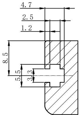
局部C 四面, M3螺母, 安装用 比例: 6: 1
